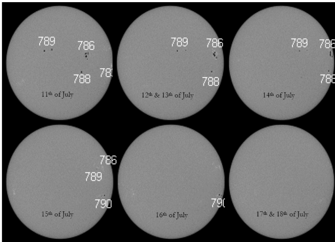
Εικόνα 1: Η εξέλιξη των ηλιακών κηλίδων από τις 11 μέχρι και τις 18 Ιουλίου 2005
