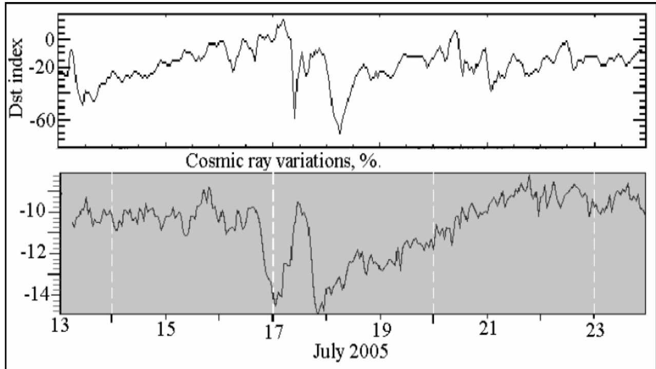
Εικόνα 3: Μεταβολές του δείκτη Dst καθώς και της έντασης της κοσμικής ακτινοβολίας όπως καταγράφηκε από τον σταθμό καταμέτρησης της Αθήνας.
